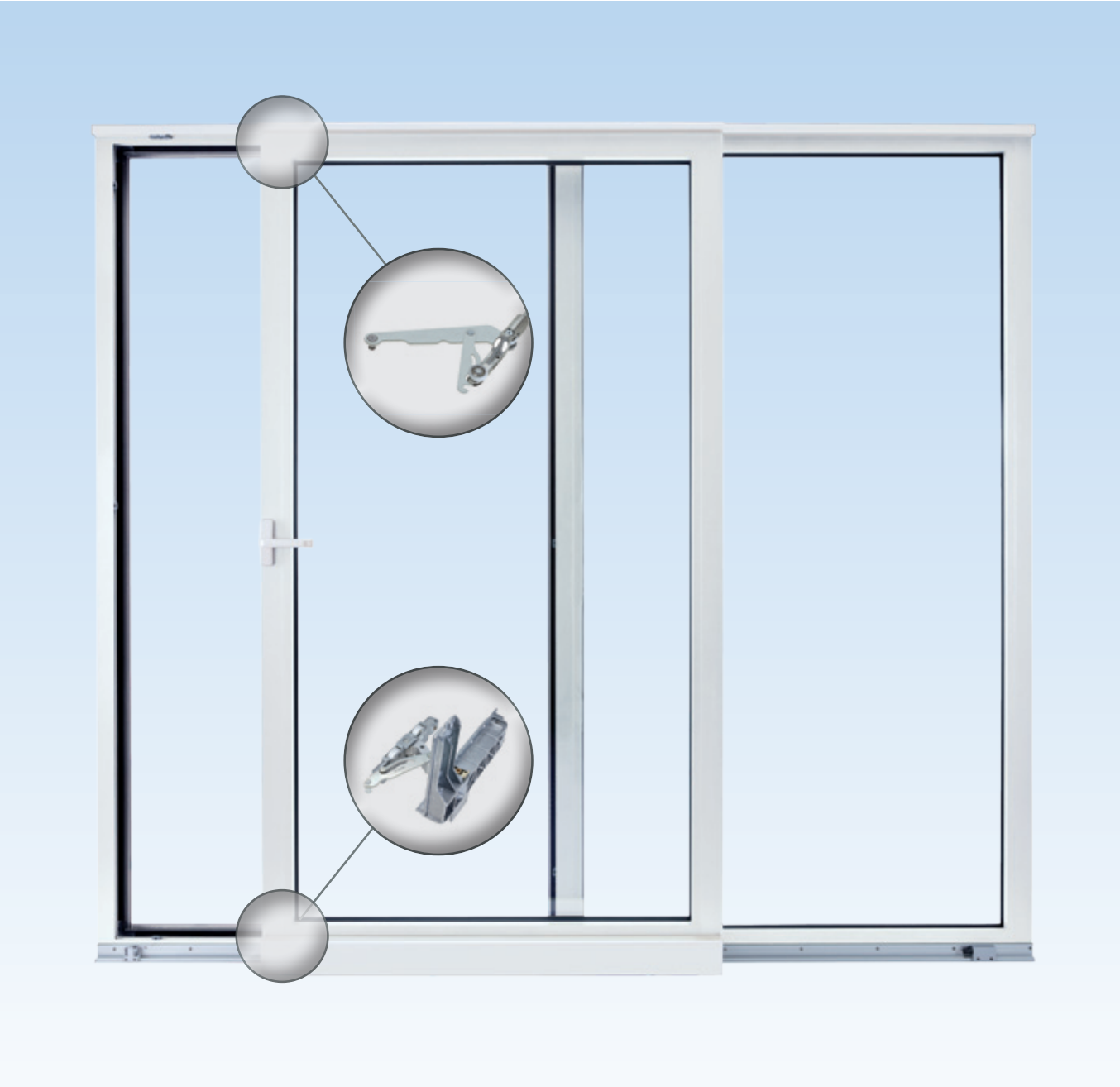
Parallelschuif-beslag GU-966/200 oZ
